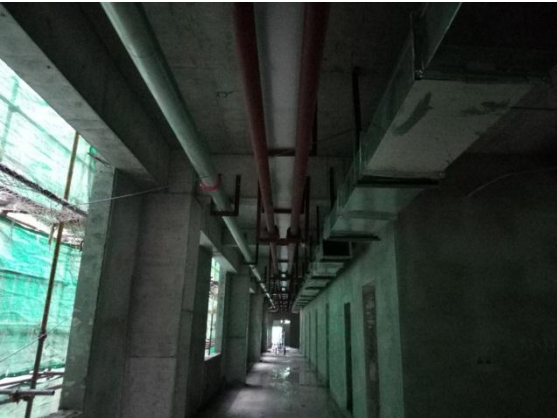
教学服务中心风管、空调水干管安装 (2017. 3. 16)
