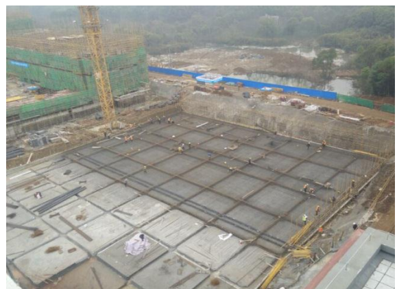
学一食堂底板钢筋绑扎 (2017.3.14)
