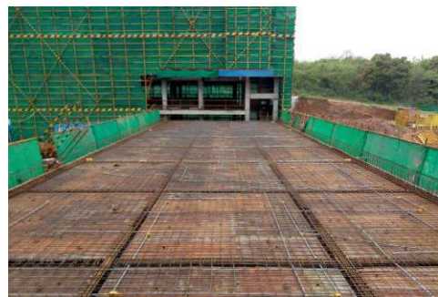
学生宿舍一组团项目 1#附属楼钢筋模板施工 (2016.4.9)
