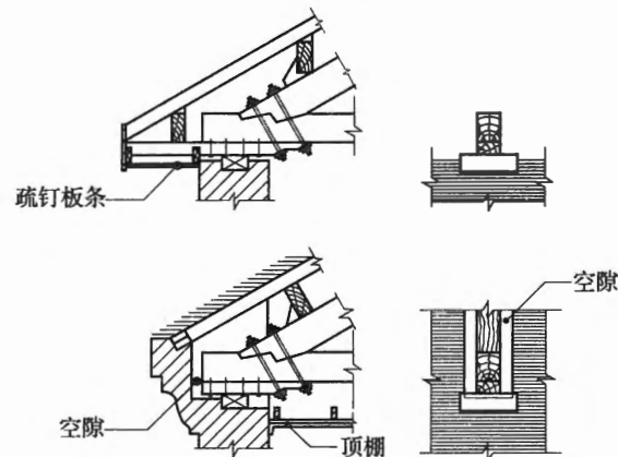
图 7.2.4-1 外排水屋盖支座节点通风构造示意
