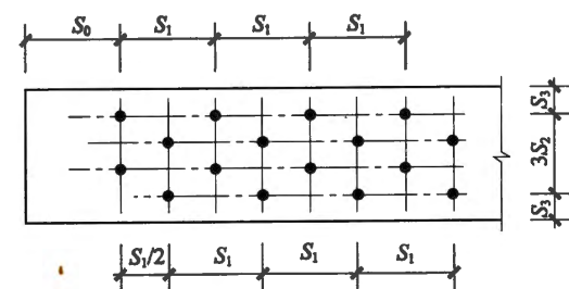
图 6.2.6-2 错列
