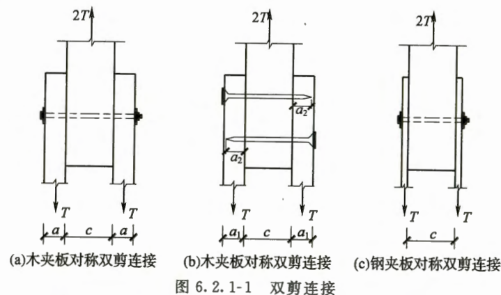
图 6.2.1-1 双剪连接
