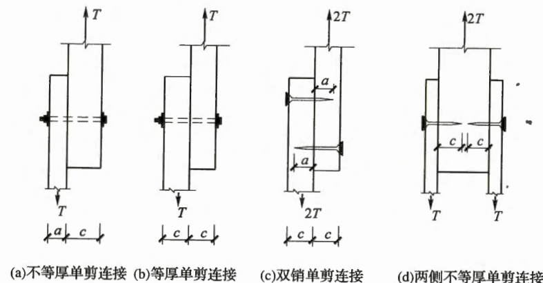
图 6.2.1-2 单剪连接
